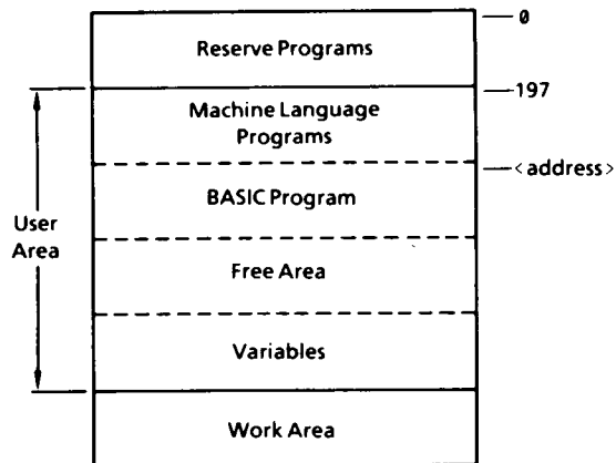
Abbildung 36: Aufteilung des Benutzer-Bereiches
