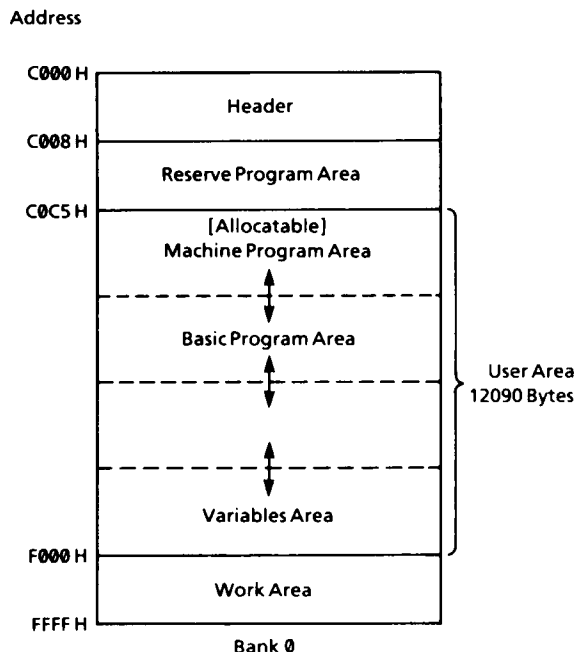
Abbildung 53 : Internes RAM
