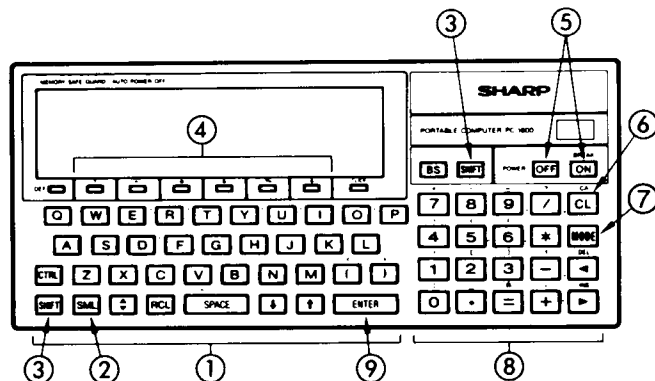
Abbildung 4 : Die Tastatur des PC-1600
