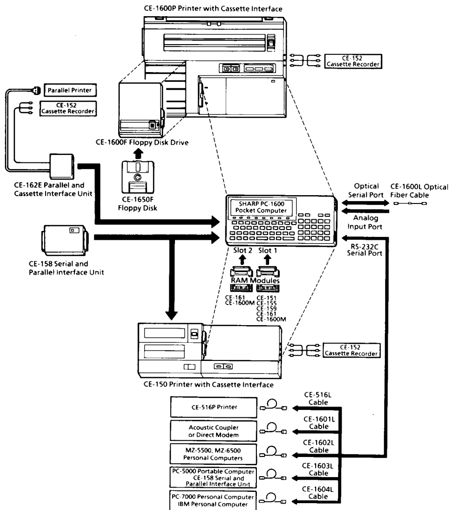
Abbildung 26 : System-Überblick
