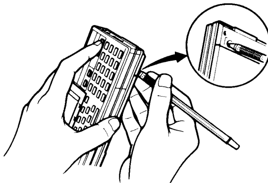
Abbildung 16 : TOTAL-RESET
