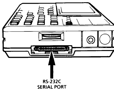
Abbildung 28 : Serieller Port
