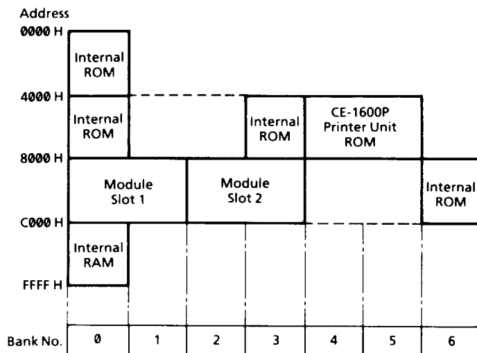
Abbildung 55 : Gesamtspeicher
