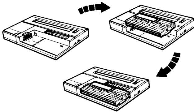
Abbildung 33 : Anschluß an den Drucker CE-1600P
