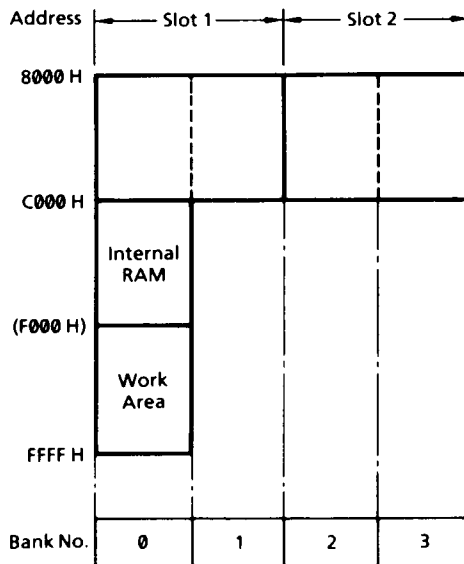
Abbildung 54 : Internes RAM und Modulfächer
